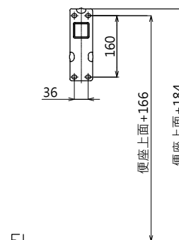
A部壁面固定螺絲位置情報
